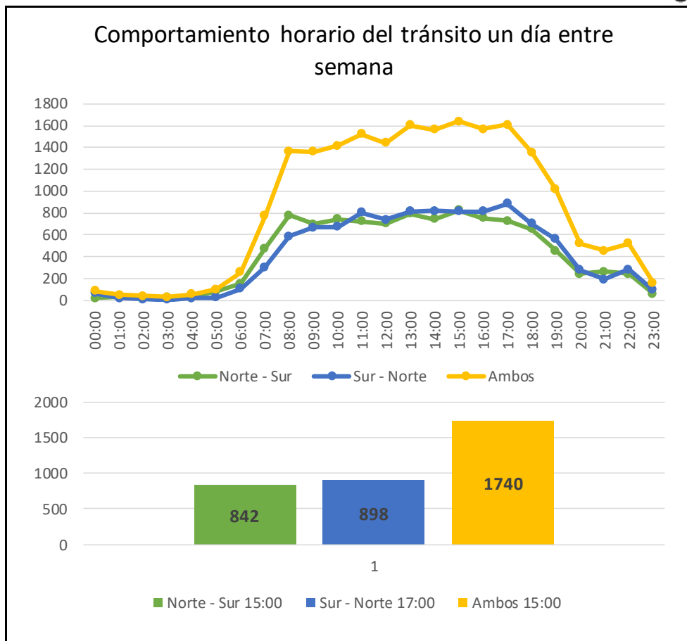
Gráfica 11.- Comportamiento horario del volumen de máxima demanda un día entre semana.
