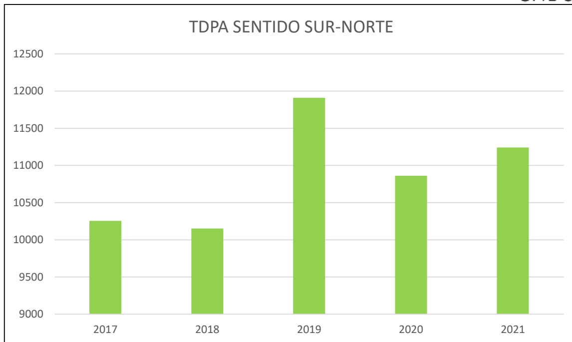
Gráfica 4.- TDPA Carretera Cuauhtémoc-Álvaro Obregón sentido Sur-Norte. Datos obtenidos de los Datos Viales de la SICT.
