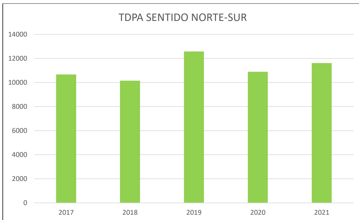
Gráfica 3.- TDPA carretera Cuauhtémoc-Álvaro Obregón sentido Norte-Sur. Datos obtenidos de los Datos Viales de la SICT.
