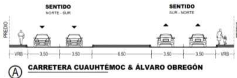
Imagen 8 Sección tipo de la carretera Cuauhtémoc-Buenaventura en el punto de instalación de equipos aforadores (km. 25)
