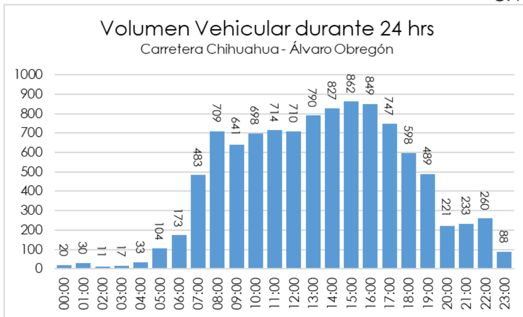
Imagen 22 Grafica de volumen vehicular durante 24 hrs.
